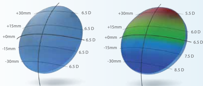
Стандардна леќа ФИКСНА БАЗНА КРИВА
