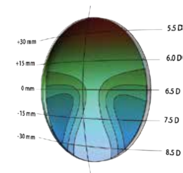
VARIA3D леќа со надворешна и внатрешна дизајнирана површина
